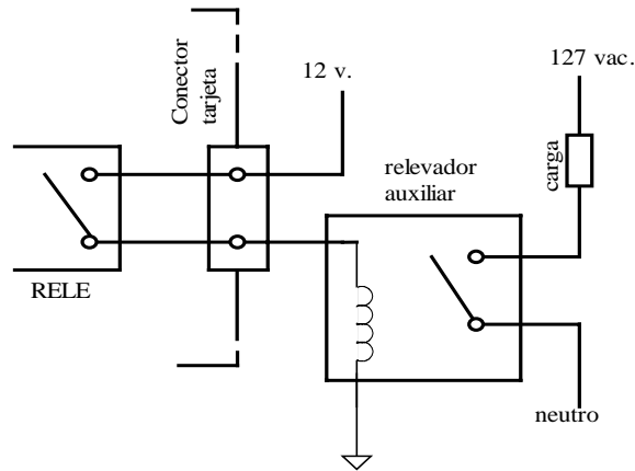
FIGURA 10: CONEXIÓN DE UN RELEVADOR AUXILIAR
